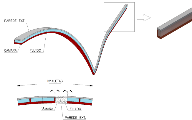
Figura 2. Simplificação da geometria.
